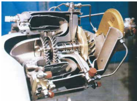
Řez generátorem vzduchu SAPHIR 5. | Foto: Archiv PBS
