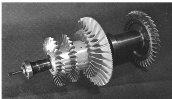
Rotor turbovrtulového motoru M 601. | Foto: Archiv PBS
