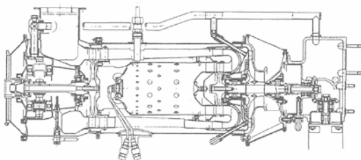
Výkres řezu turbostartérem Ts – L-39 | Foto: Archiv PBS
