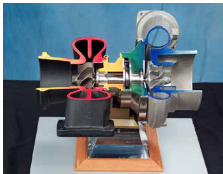
Turbodmychadlo s radiální turbínou. | Foto: Archiv PBS
