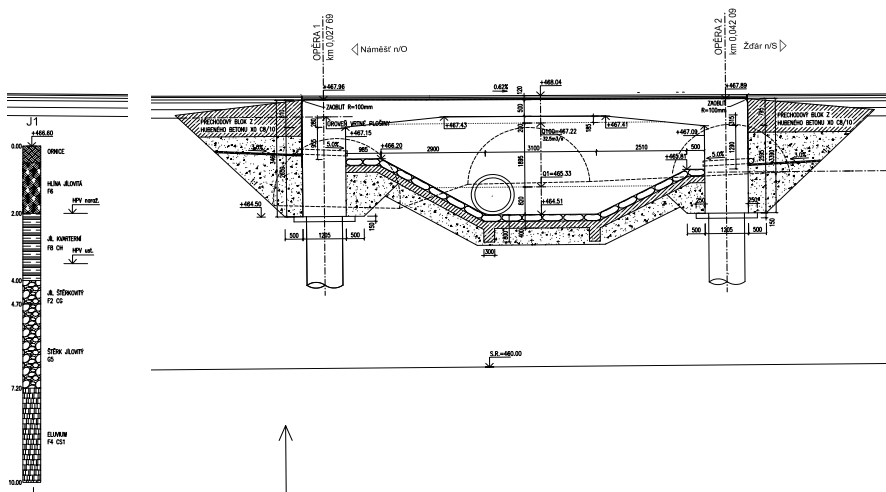
Projekt mostu – boční řez
